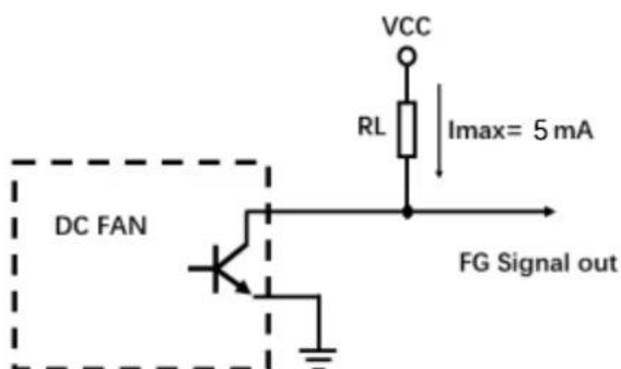
原理图
