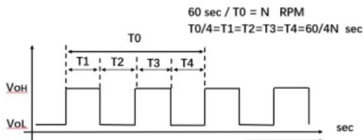
FG信号波形
