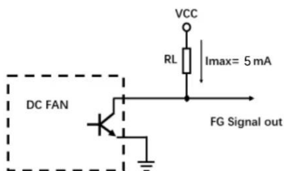
原理图
